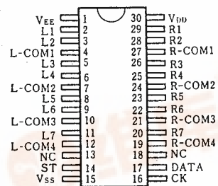
NJU7311AM
