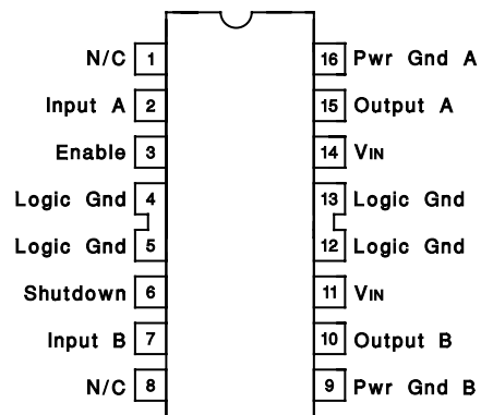
DIL-16 (Top View) JE or NE Package
