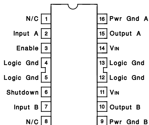
DIL-16 (Top View) JE or NE Package
