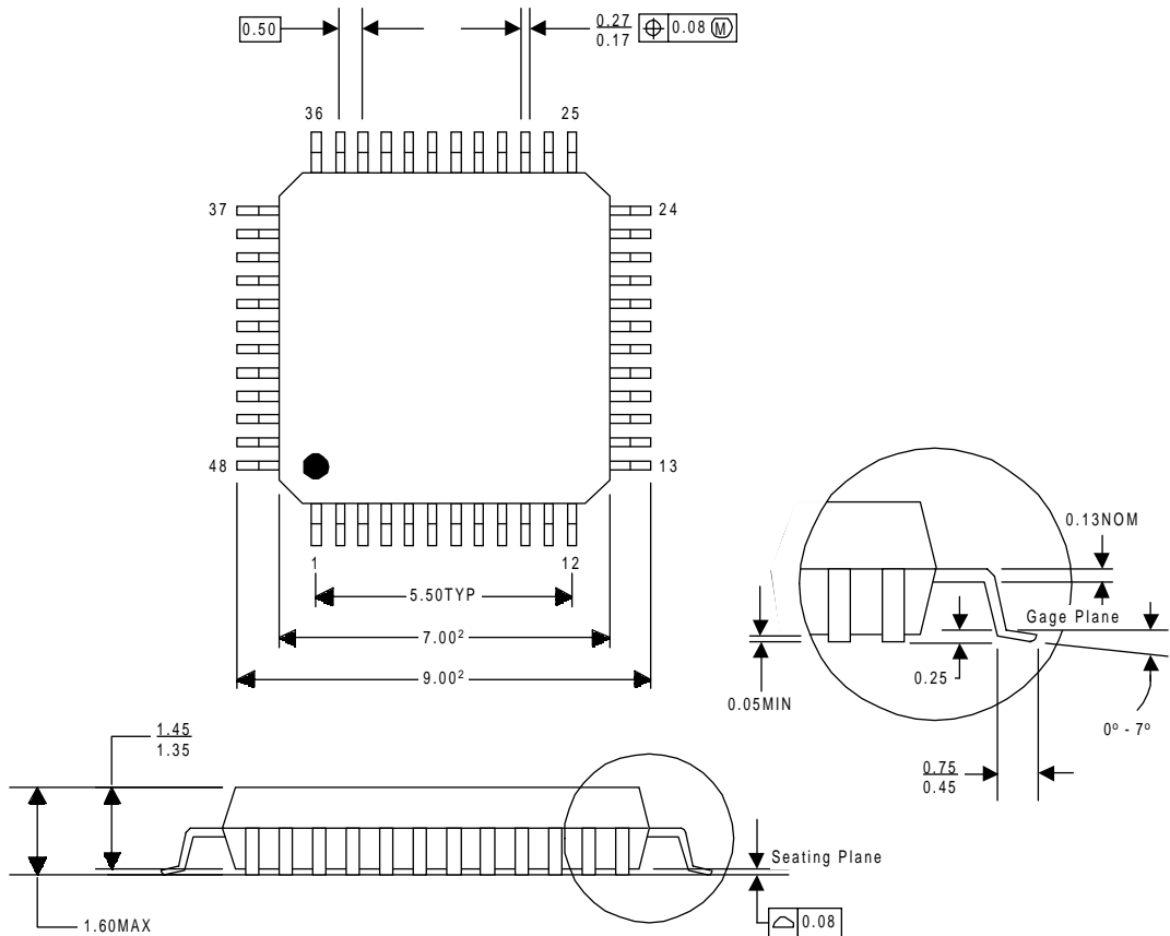
48 Pin TQFP
