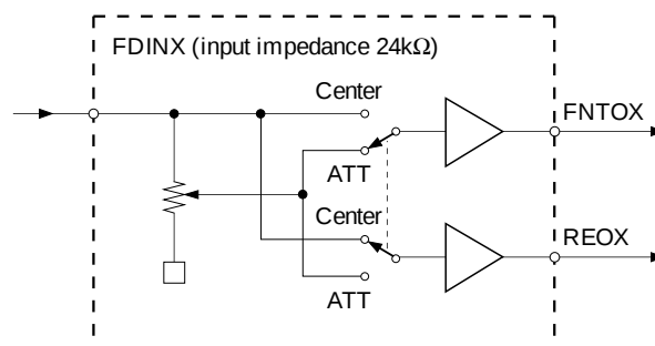
Fig. 7. Fader
