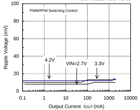
FOSC=300kHz, V_{OUT}=1.2V
