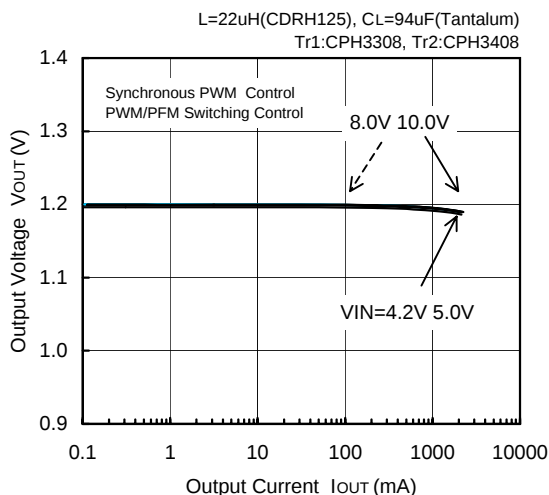
FOSC=300kHz, V_{OUT}=1.2V
