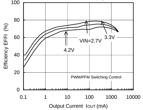
FOSC=300kHz, V_{OUT}=1.2V
