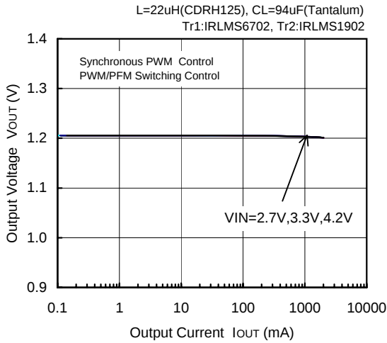
FOSC=300kHz, V_{OUT}=1.2V
