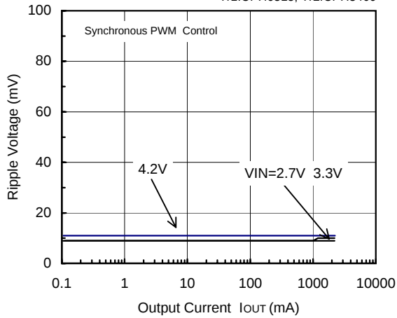
FOSC=300kHz, V_{OUT}=1.2V
