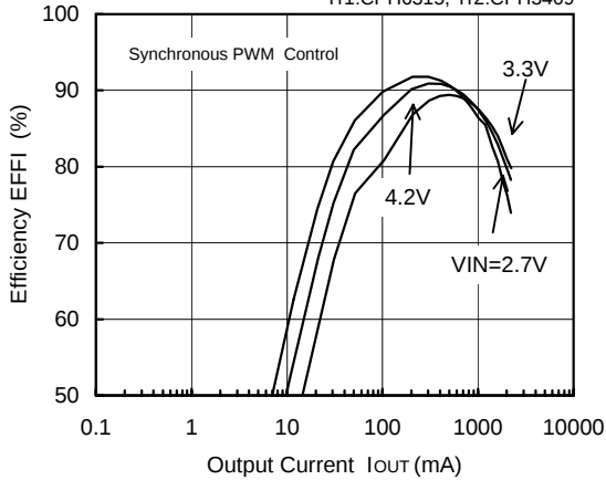
FOSC=300kHz, V_{OUT}=1.2V
