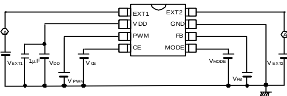
Circuit 1 :
