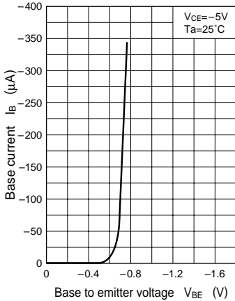
I_B - V_{BE}
