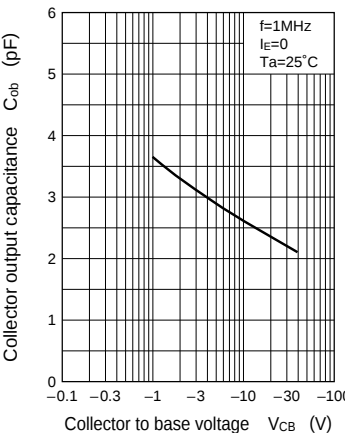
C_{ob} - V_{CB}
