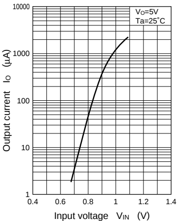
I_O - V_{IN}
