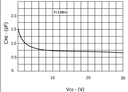
C_{RE} v V_{CE}
