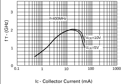
f_T v I_C
