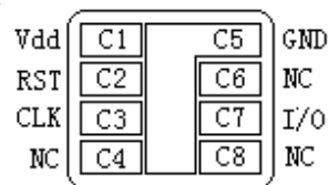
图 1 管脚图
