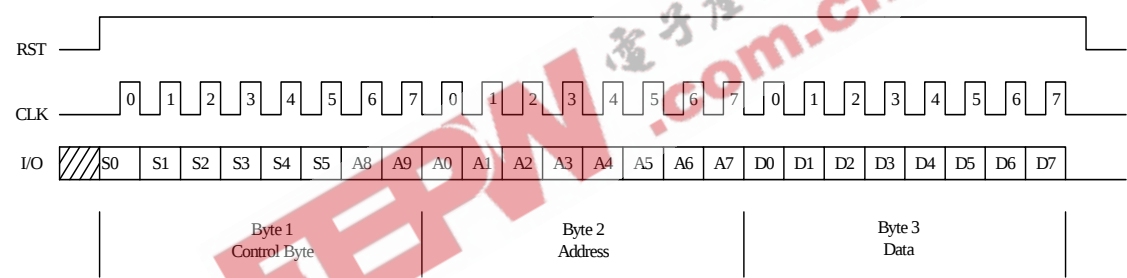
图 4 命令输入时序图
