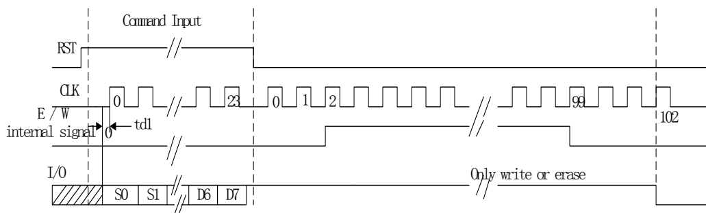
图 6 只写、只擦时序
