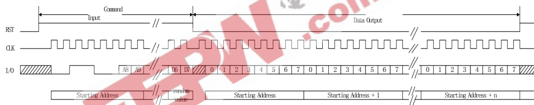
图 7 读数据字节时序
