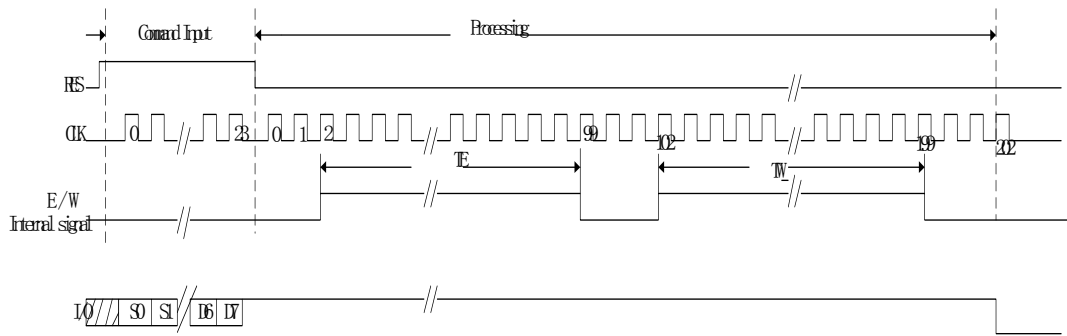
图 5 擦除并写入时序
