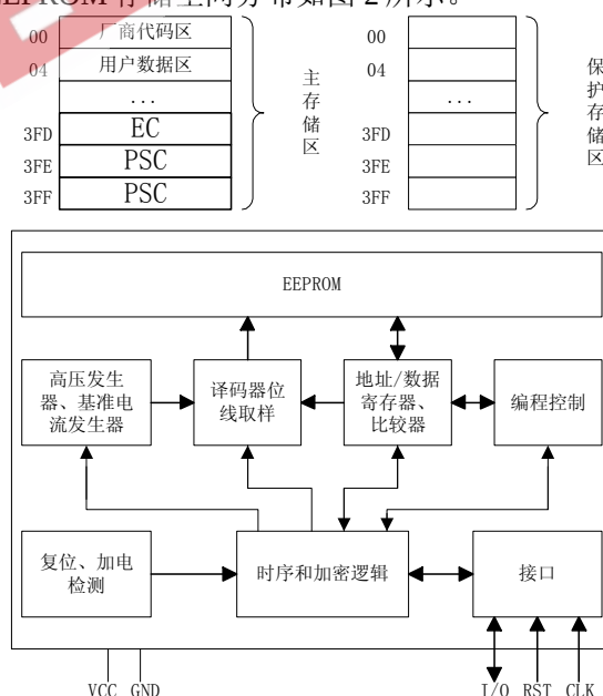
图 2 电路框图和存储空间分布
