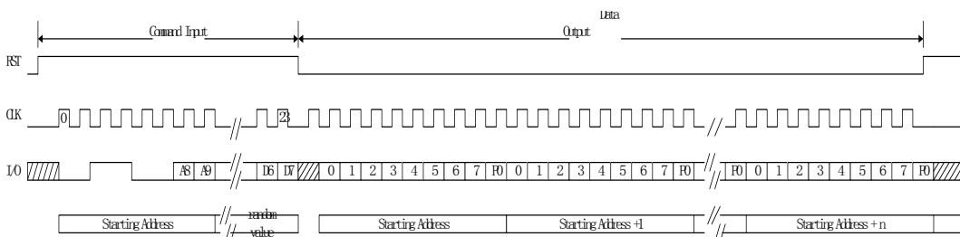
图 8 读数据字节包括保护位时序
