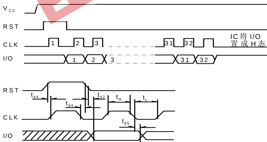
图 3 复位和应答复位
