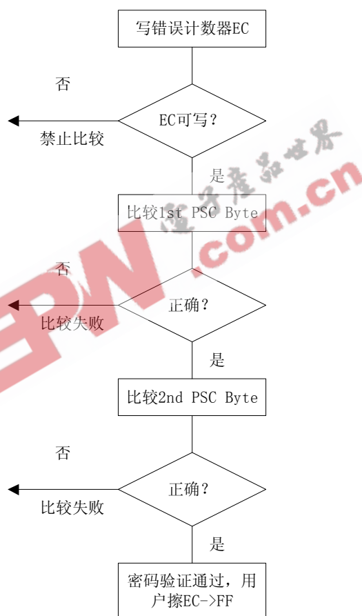
图 9 密码验证流程
