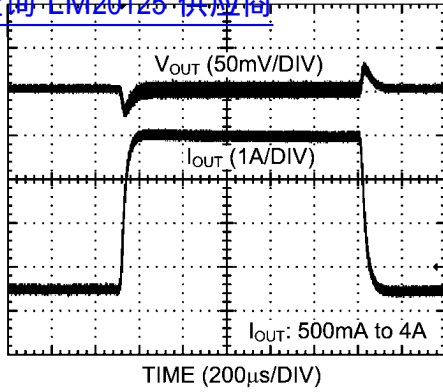
Load Transient Response 查询"LM20125"供应商
