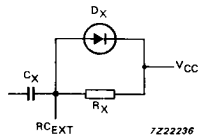
Fig. 11 Power-down protection circuit.
