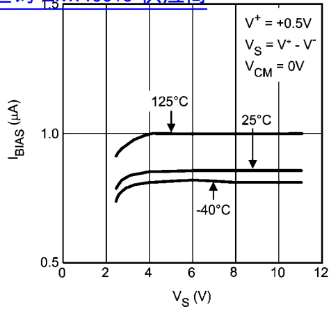
I_B vs. V_S (npn) 查询"LMH6618"供应商
