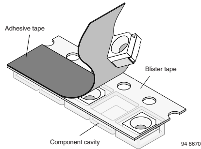
Fig. 10 - Blister Tape
