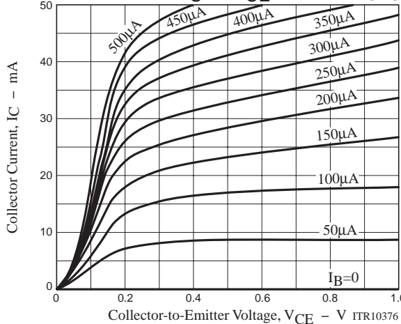
I_C - V_{CE} [TR]
