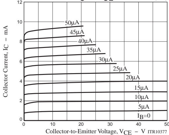
I_C - V_{CE} [TR]
