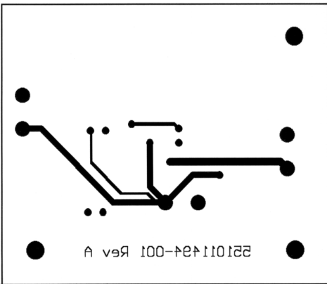
Bottom Layer
