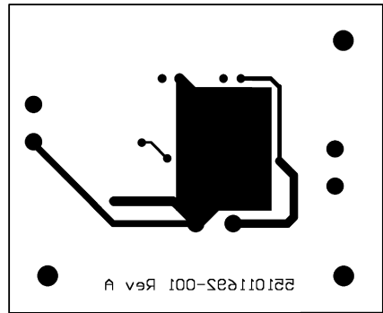
Bottom Layer
