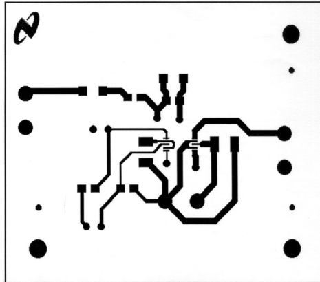
Top Layer
