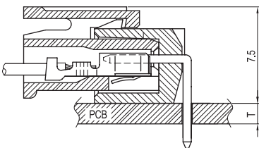
PCB ASS'Y
