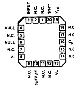
SMP-11BRC/883 LCC PACKAGE (RC-Suffix)
