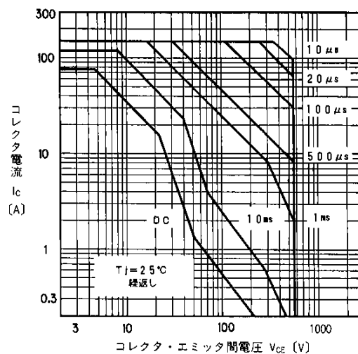
安全動作領域特性(繰返し)
