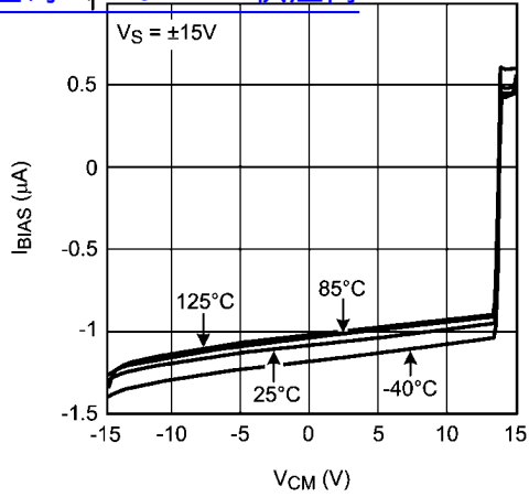
I_{BIAS} vs. V_{CM} 查询"LM7321MA"供应商
