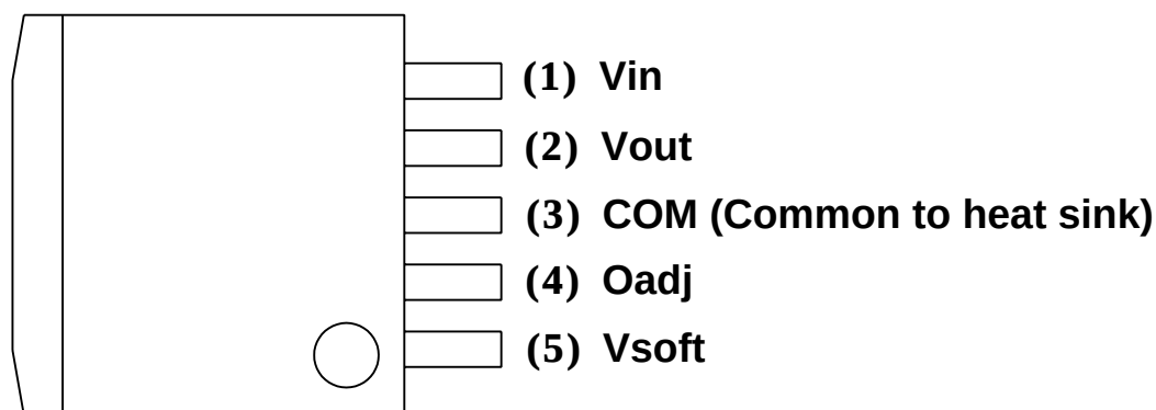
(TO-263-5)
