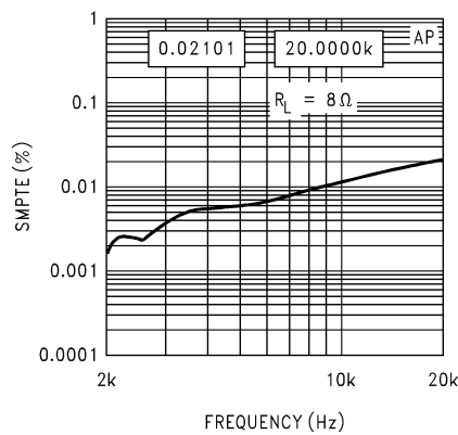
IMD 60 Hz, 1:1
