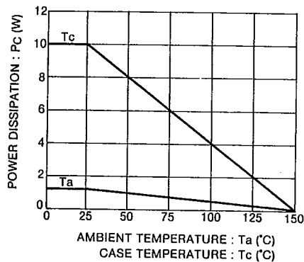
Fig.1 電力軽減曲线
