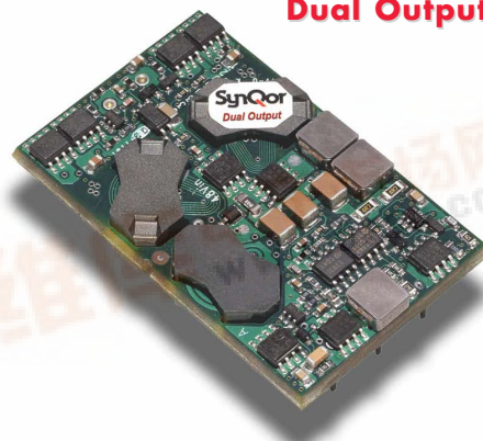
DQ65033QMA06 Module
