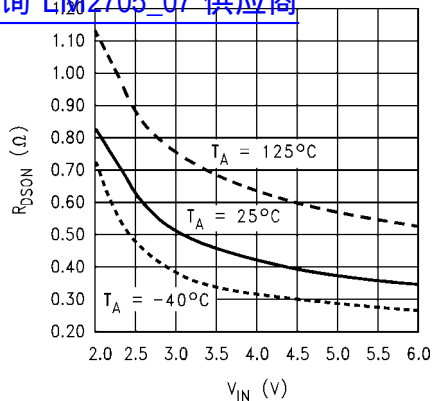
Switch R_{DS(on)} vs V_{IN} 查询"LM2705-07"供应商
