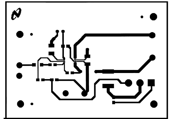
Top Layer
