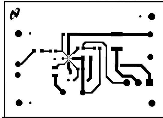
Top Layer
