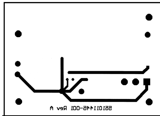
Bottom Layer
