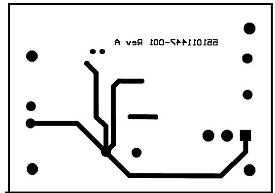
Bottom Layer
