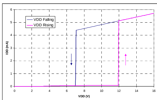
Figure 5a: I DD vs. V DD (V DD_ON )
