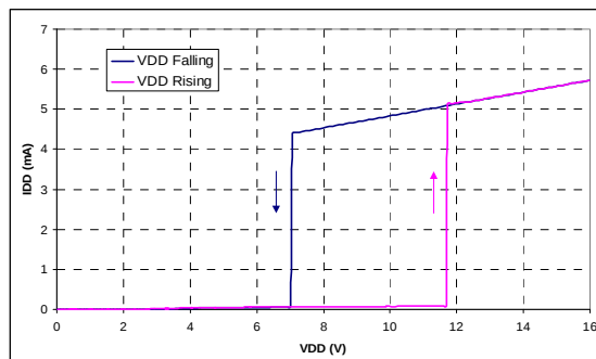
Figure 5b: I DD vs. V DD (V DD_ON )
