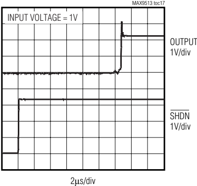
ENABLE TIME
