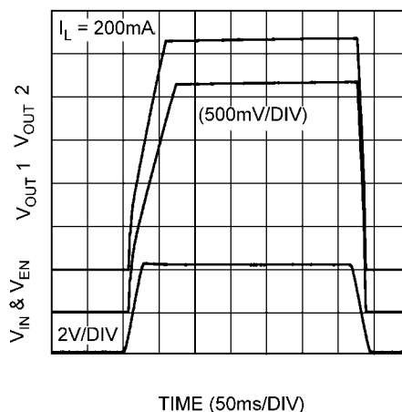
Vin and Enable Tied Together
