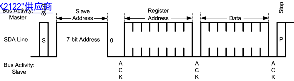
FIGURE 20. Write Byte
