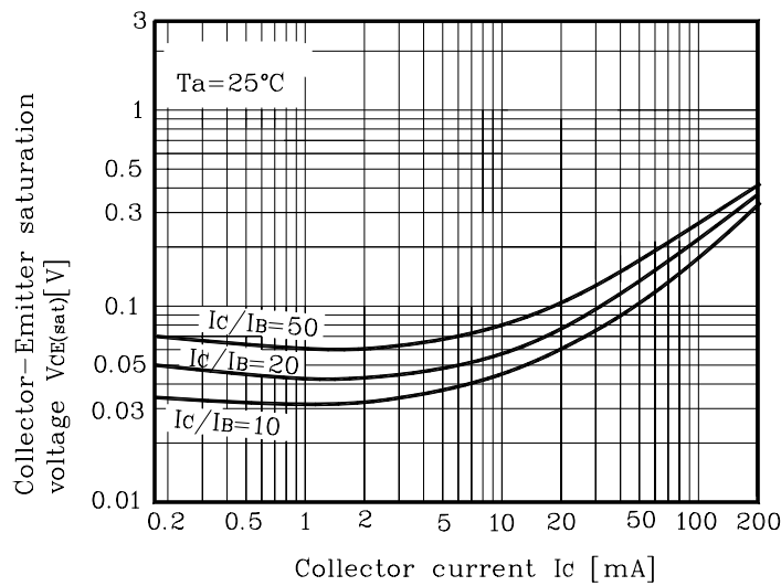
Fig. 5 V_{CE(sat)} - I_C
