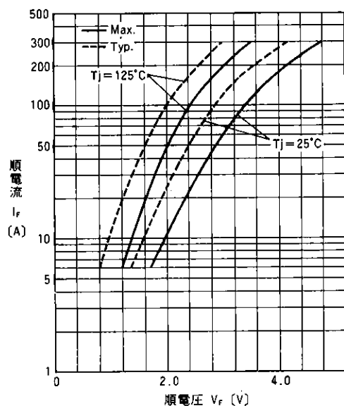
順特性
