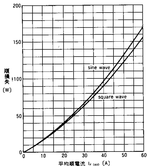
順損失
