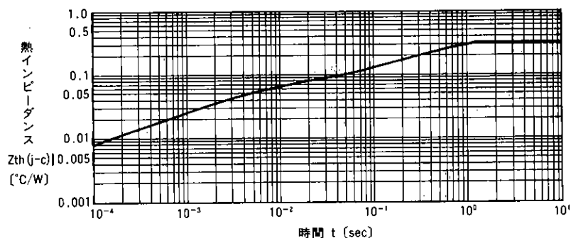
過渡熱インピーダンス
