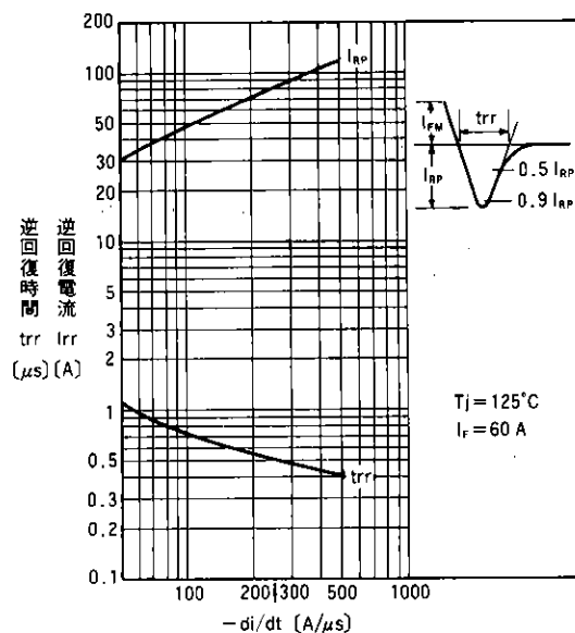
逆回復特性
