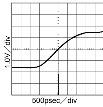
Fig.22 VCXO_OUT(27MHz) Period-Jitter VDD=3.3V,CL=4pF
