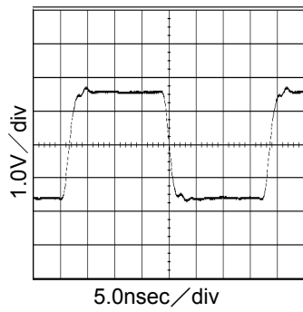
Fig.21 VCXO_OUT(27MHz) output waveform VDD=3.3V,CL=4pF
