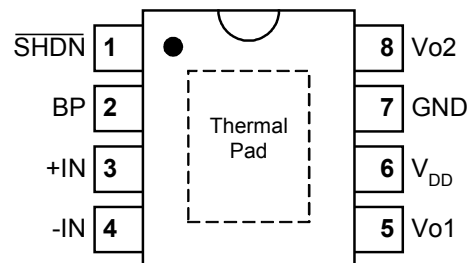
SOP8, MSOP8
