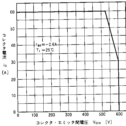
コレクタ電流 I_c (A) 安全動作領域(逆バイアス) Reverse Biased Safe Operating Area
