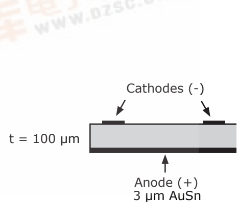
Die Cross Section
