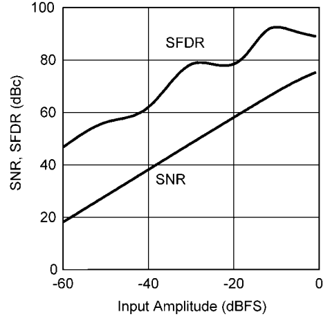
SNR, SFDR vs. Input Amplitude (dBc)
