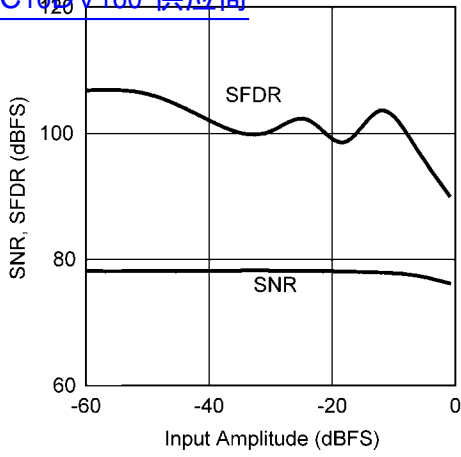
SNR, SFDR vs. Input Amplitude (dBFS) 查询"ADC16DV160"供应商
