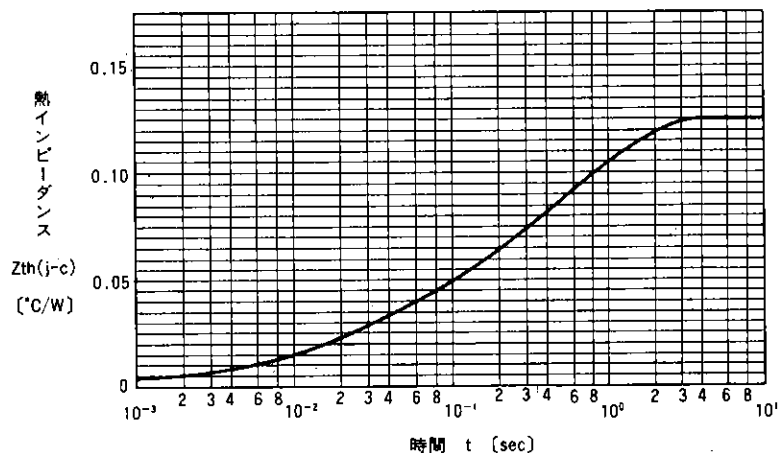
過渡熱インピーダンス
