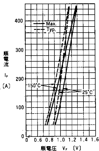
順特性
