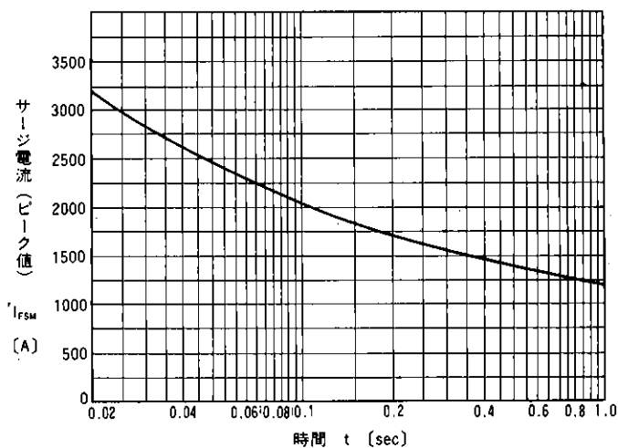
サージ電流
