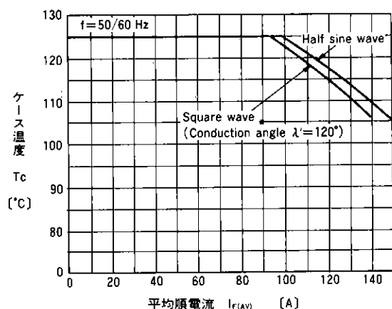
ケース温度—平均出力電流
