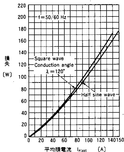
総損失—出力電流
