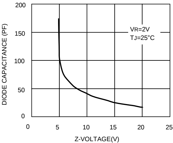
FIG.6 - DIODE CAPACITANCE VS.Z-VOLTAGE
