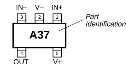
SOT-23-5 or SC-70
