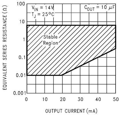
LM2936-5.0 C OUT ESR
