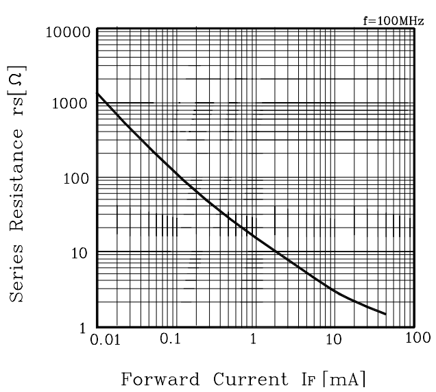
Fig. 4 r_s - I_F
