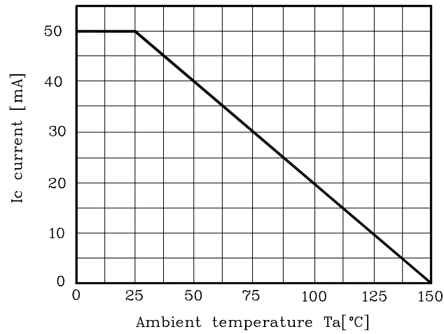
Fig. 1 I_C - T_a
