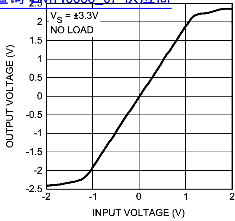
查询"LMH6583_07"供应商 No Load Output Swing
