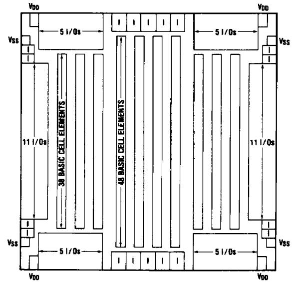
6212 Die Structure
