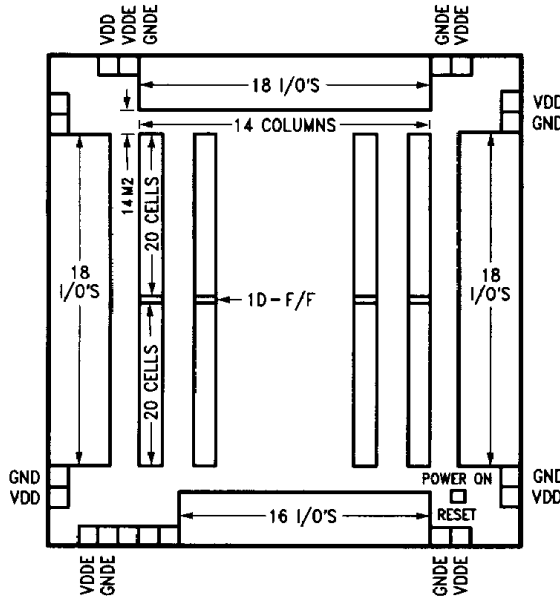
6218 Die Structure
