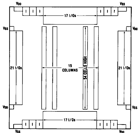
6225 Die Structure
