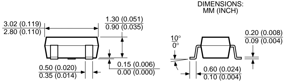
SOT-23-5 (M)
