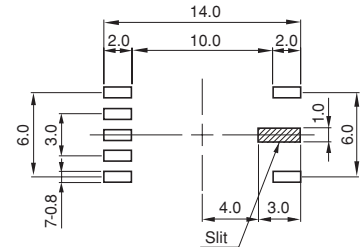
LAND PATTERNS (mm) 推奨ランド寸法
