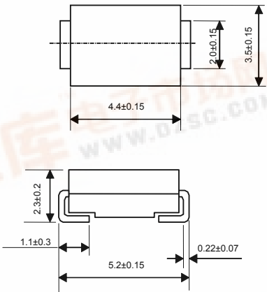
SMB / DO-214AA
