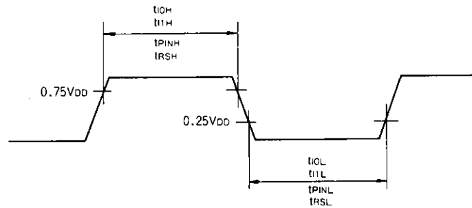
Fig. 7 \text{INT0} , \text{INT1} , \text{INT2} , \text{INT3} , \text{INT4} , \text{INT5} , \text{PIN1} , \overline{\text{RES}} Input Timing
