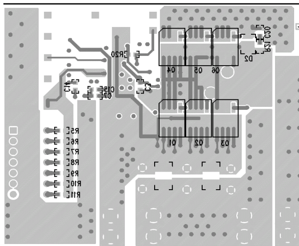
Figure 33. Bottom layer
