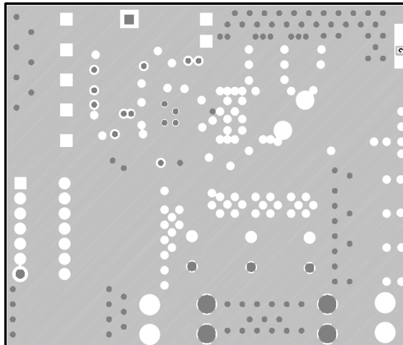
Figure 33. Bottom layer
